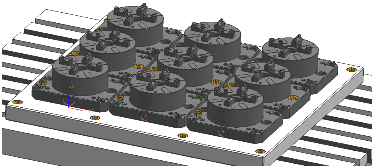
9-fach mit manuellem Ventil auf Aluminiumplatte
