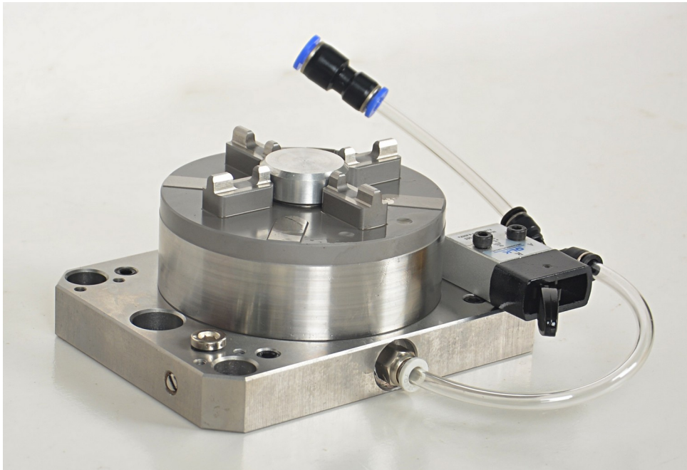
Cfg. 1 Direct air connection with valve switch (4 possible mounting options) Direkt per Luftanschluss mit Pneumatikschalter (4 Positionen möglich)
