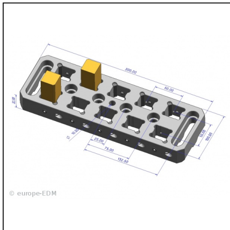
Leiste mit 10-fach Vierkant 25mm Spannsystem
