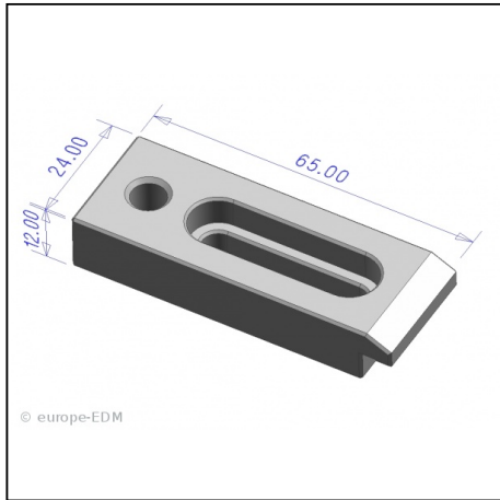
Spannpratze Länge 65mm für Drahtschneideleiste
